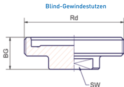
Blind-Gewindestutzen
