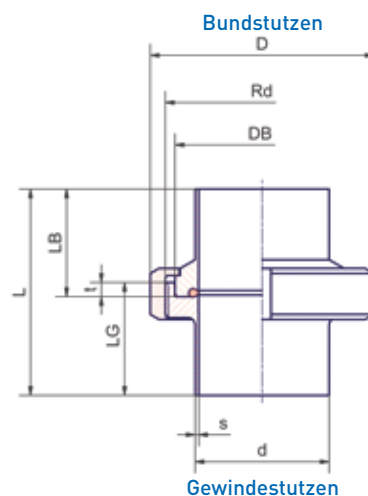
Gewindestutzen
