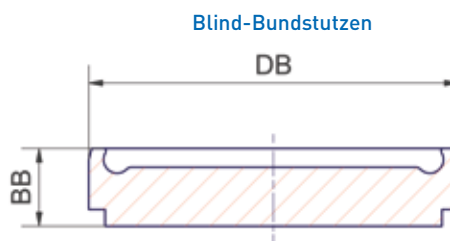
Blind-Bundstutzen
